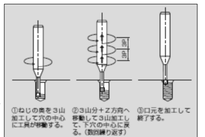
図3 プラネットカッタによる加工方法
